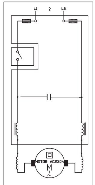
ESQUEMA ELECTRICO 230 V.
